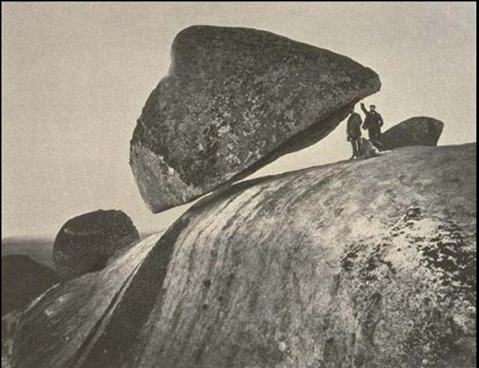
Piedra movediza del Tandil - Argentina
